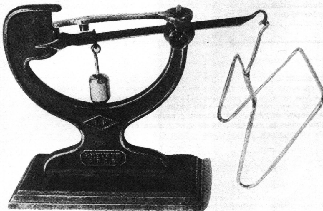
Un curieux pèse-lettre (voir page 807 de ce numéro)
